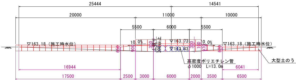
断面図 S=150
