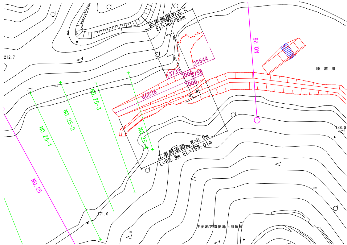
平面図 S=1000
