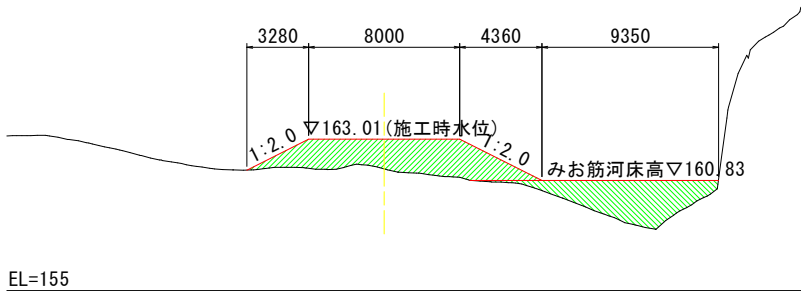
A-A断面
