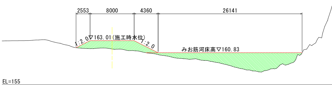
B-B断面
